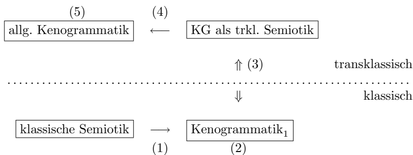
Abbildung 3.7: Kenogrammatik und Semiotik
