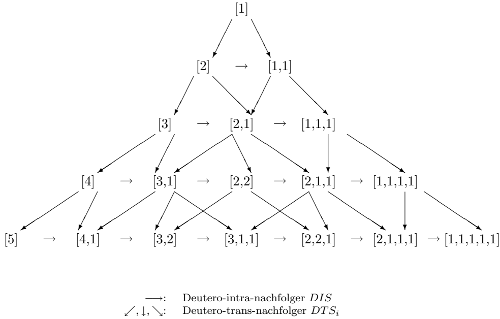
Abbildung 4.4: Die ersten fünf Deuterocontexturen als Partitionen
