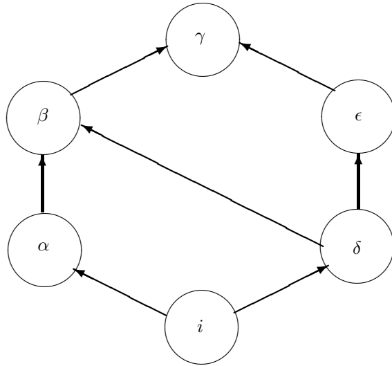
Abbildung 3.8: Das Verhältnis der sechs Charakteristika nach Schadach. Die Pfeile \longrightarrow symbolisieren die Implizierungsrelation.
