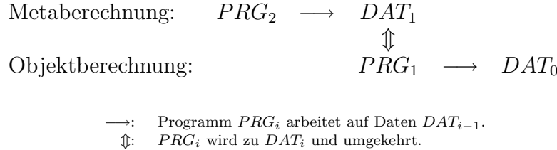
Abbildung 10.6: Logische Ebenen einer reflektiven Berechnung
