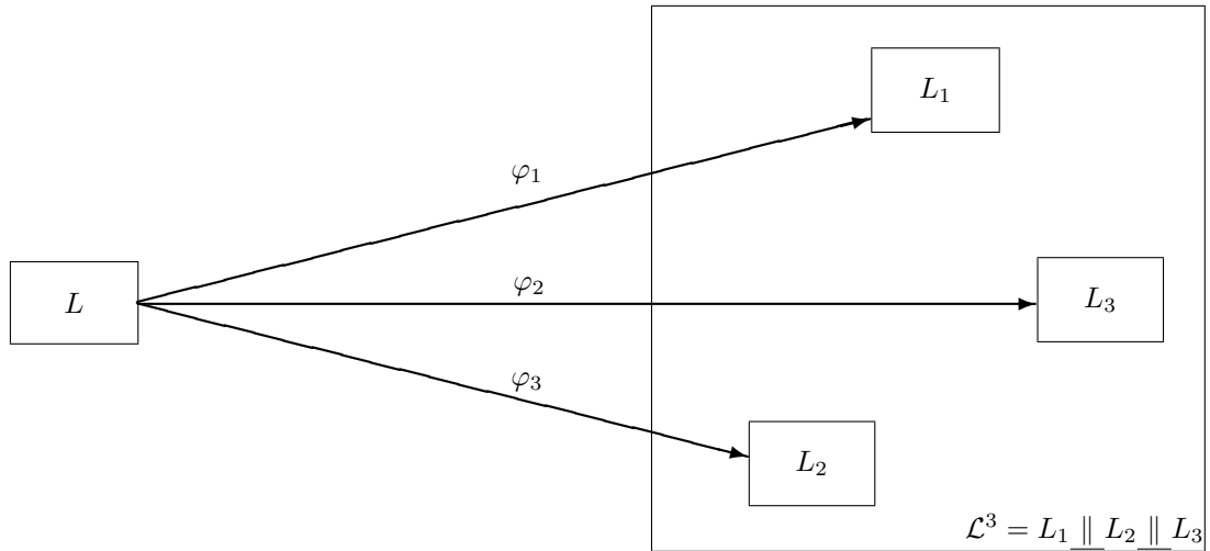
Abbildung 9.1: Distribution der klassischen Logik über mehrere Kontexturen als Fasersraum
