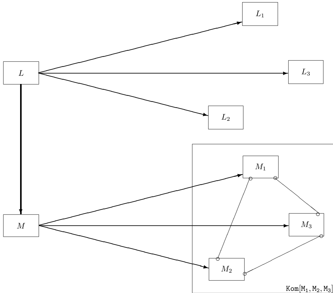
Abbildung 9.3: Morphogrammatische Komposition von Verbundstrukturen. \circ\text{---}\circ stellt dabei die Vermittlung der Subsysteme gemäß \equiv_{VB} dar.
